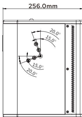
HQ1000/HQ1000W侧面
