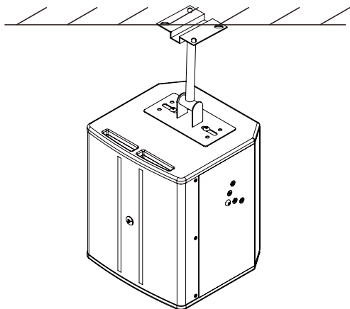
顶部吊挂图
