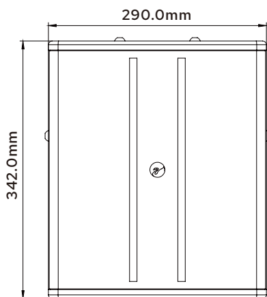
HQ1000/HQ1000W正面
