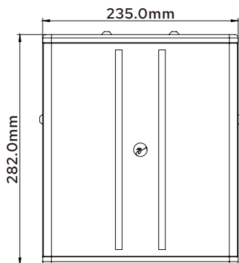
HQ1000/HQ1000W正面
