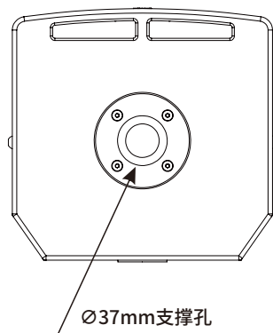
底面
