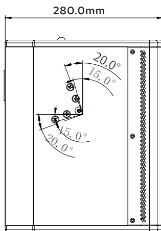
HQ1000/HQ1000W侧面
